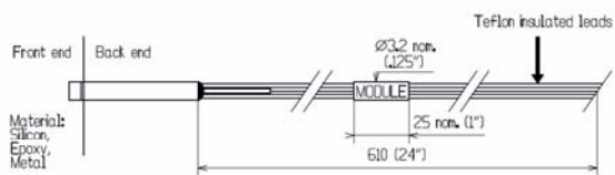
WIRING – EXTERNAL MODULE
